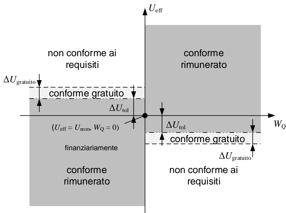
Figura 1: Principio di conformità per il ruolo attivo. U_{\text{eff}} è la tensione effettiva, U_{\text{nom}} è la tensione nominale sul nodo elettrico della rete di trasmissione. \Delta U_{\text{tol}} è la tolleranza applicata nel conteggio e \Delta U_{\text{gratuito}} è la fascia liberamente conforme. W_Q è lo scambio netto di energia reattiva nel corrispondente quarto d'ora. Sinistra: comportamento come capacità (fornitura di energia reattiva alla rete di trasmissione); destra: comportamento come induttanza (prelievo di energia reattiva dalla rete di trasmissione).
